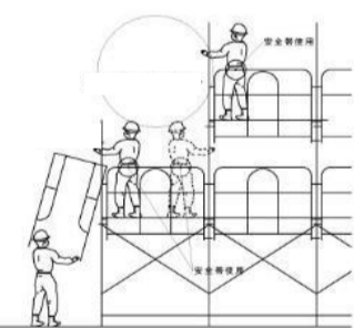
枠組足場
